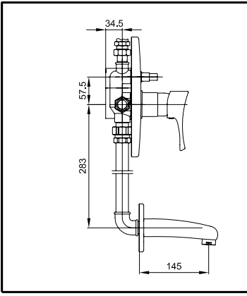
YARI ANKASTRE BANYO BATARYASI 102102364
