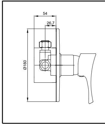
ANKASTRE DUŞ BATARYASI 102102365
